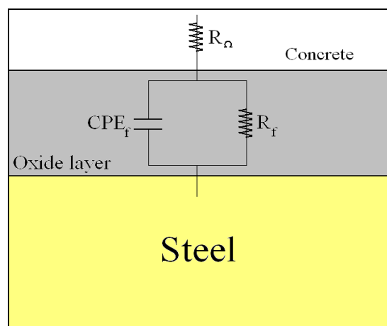
شکل (۹): مدار معادل الکتریکی فولاد در بتن در شرایطی که لایه ای بر روی فولاد تشکیل شده است.
