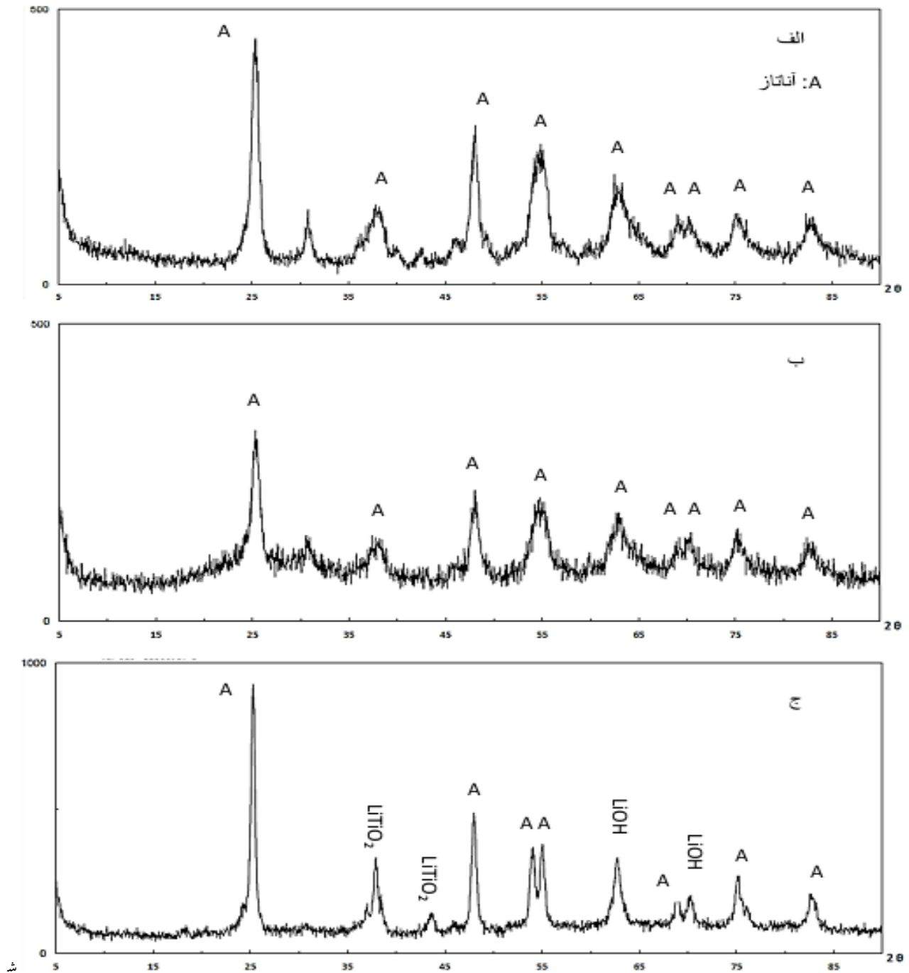
شکل (۱): الگوی XRD مربوط به پودرهای TiO_2 دوپ شده با: (الف) ۰/۳۶، (ب) ۰/۷ و (ج) ۱/۱۴ درصد وزنی لیتیوم.
