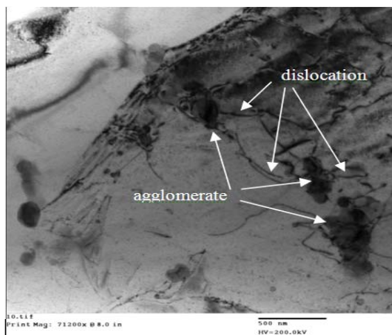
شکل (۶): تصویر TEM از ریزساختار نمونه Mix پس از آزمون کشش که نشان‌دهنده قفل شدن نابجایی‌ها در اطراف ذرات و آگلومرها می‌باشد.
