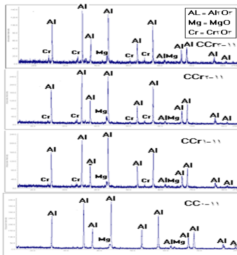
شکل (۴): الگوی پراش اشعه ایکس در نمونه CCr0-11 و نمونه‌های CCr1-11 ، CCr2-11 ، CCr3-11 .
