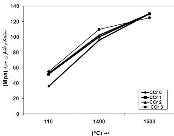
شکل (۳): نمودار استحکام فشاری سرد بر حسب دما.
