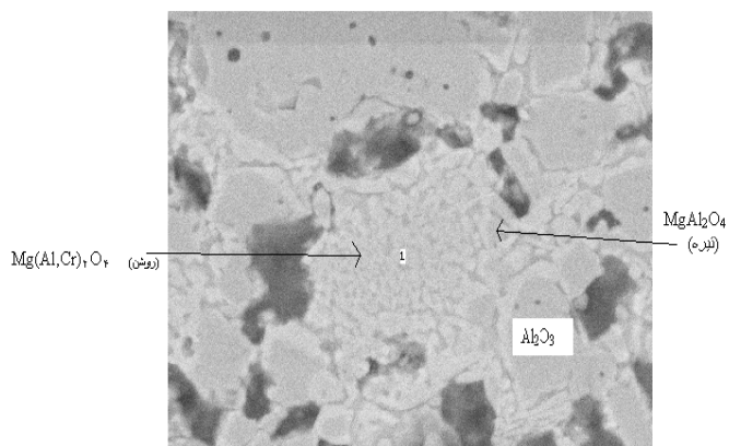
شکل (۹): ریزساختار نمونه ۱۴-CCr۱۳ با بزرگنمایی ۱۵۰۰
