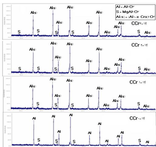
شکل (۵): الگوی پراش اشعه x نمونه CCr1-14 و نمونه‌های CCr2-14 ، CCr3-14 ، CCr4-14 .
