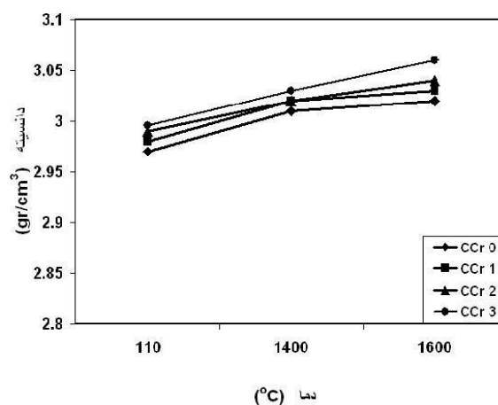
شکل (۱): نمودار دانسیته بر حسب دما.
