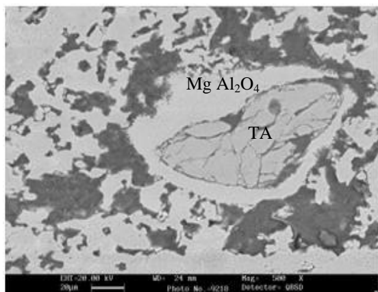
شکل (۸): ریزساختار نمونه ۱۴-CCr۰ در بزرگنمایی ۵۰۰
