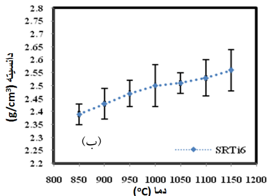
شکل (۳): تغییرات (الف) درصد انقباض خطی، (ب) چگالی شیشه‌سرامیک حاوی ۶ درصد وزنی TiO_2
