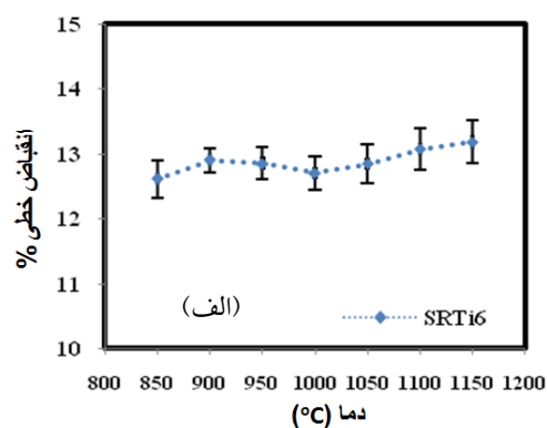
شکل (۳): تغییرات (الف) درصد انقباض خطی، (ب) چگالی شیشه‌سرامیک حاوی ۶ درصد وزنی TiO_2
