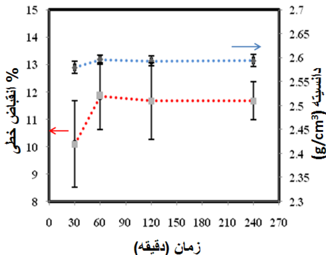
شکل (۵): تغییرات چگالی و انقباض خطی شیشه سرامیک SRTi6 عملیات حرارتی شده در دمای 1150^\circ\text{C} و زمان‌های نگهداری مختلف
