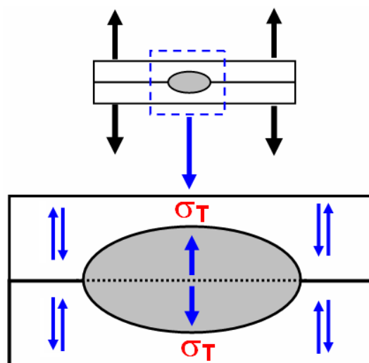
شکل (۹): یک مدل ساده از توزیع تنش در فصل مشترک و محیط دکه جوش در آزمون کشش متقاطع
