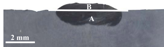
شکل (۲): مقطع عرضی از موضع روکش کاری شده A و B به ترتیب مشارکت زیرلایه و فلز پرن در لایه روکش
