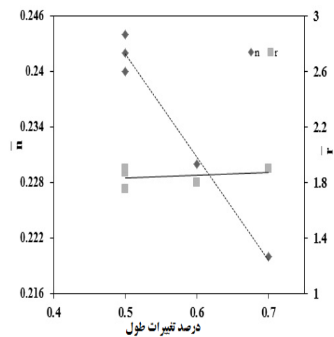
شکل (۸): ارتباط درصد تغییرات طول نورد پوسته‌ای بر اساس \bar{r} و \bar{n}
