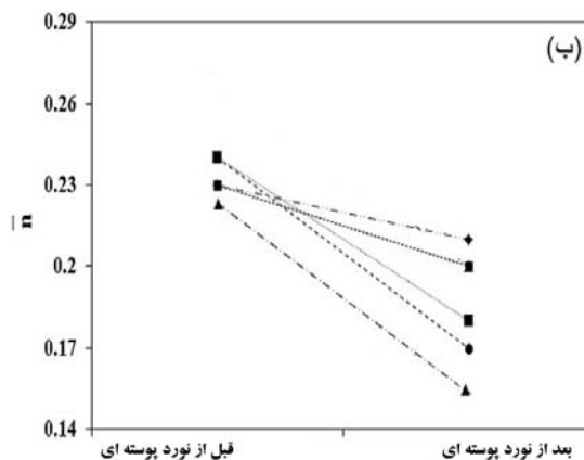
شکل (۳): تغییرات (الف) \bar{\Gamma} و (ب) \bar{n} برای مجموعه (A) قبل و بعد از نورد پوسته‌ای
