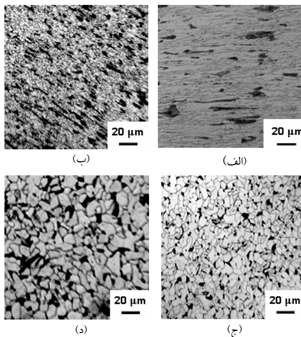
شکل (۳): ریزساختار فولاد مورد آزمون با تغییر شکل در دمای محیط با کرنش ۲/۵، (الف) در حالت تغییر شکل یافته و آئیل شده در دمای آئیل ۴۰۰°C و زمان آئیل، (ب) ۱ دقیقه، (ج) ۵ دقیقه و (د) ۳۰ دقیقه.
