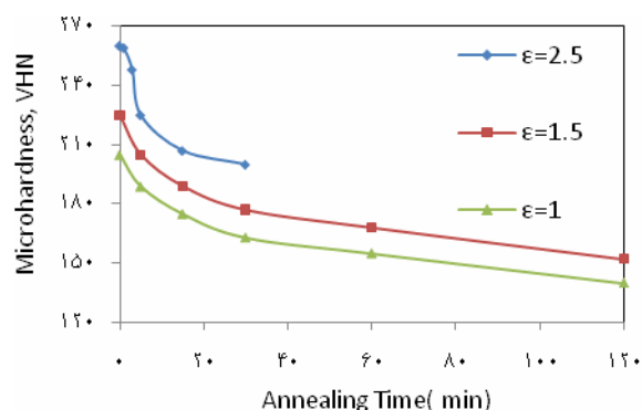
شکل (۷): تغییرات ریزسختی فولاد مورد آزمون بر حسب زمان آنیل در دمای آنیل ۴۰۰°C و مقادیر مختلف کرنش.
