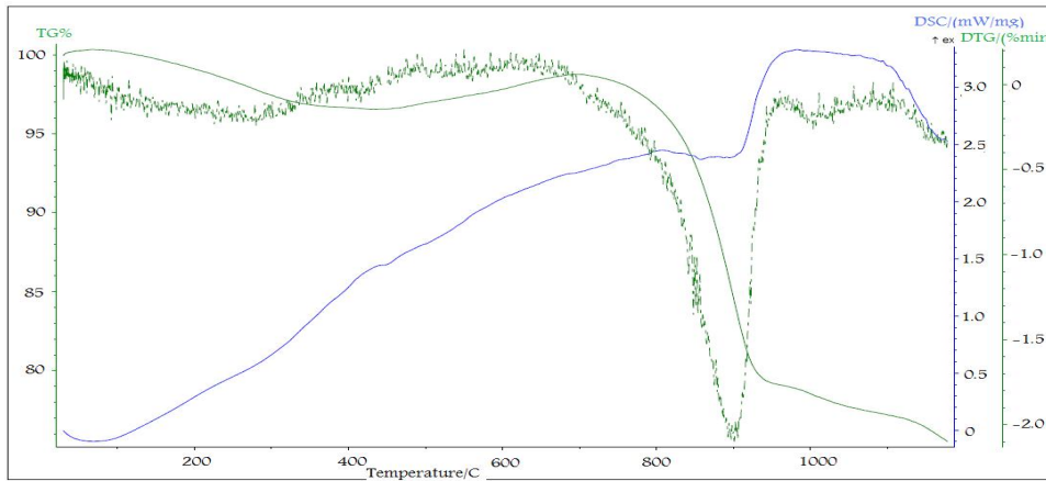
شکل (۳): منحنی‌های TG-DSC برای مخلوط کنسانتره و آهک فعال‌سازی شده به مدت زمان ۱۰ ساعت تحت اتمسفر اکسیژن.
