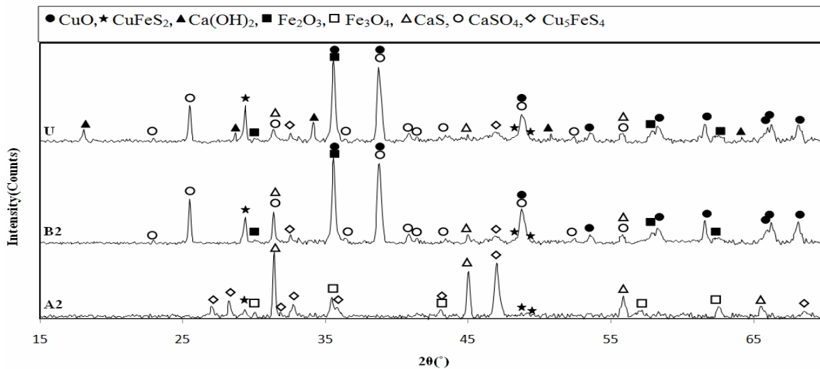
شکل (۴): الگوهای پراش پرتو ایکس نمونه‌های تشویه شده در اتمسفرهای آرگون و هوا (U) نمونه فعال‌سازی نشده و تشویه شده در هوا، B 2 : نمونه فعال شده و تشویه شده در هوا و A 2 : تشویه شده در هوا و تشویه شده در محیط آرگون.
