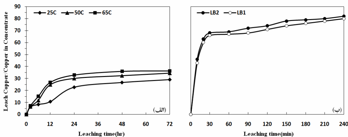
شکل (۵): نمودارهای تغییرات بازیابی مس بر حسب زمان فروشویی برای نمونه‌های (الف): کنسانتره فعال‌سازی نشده و (ب): اکتیو شده مکانیکی LB2 و LB1.
