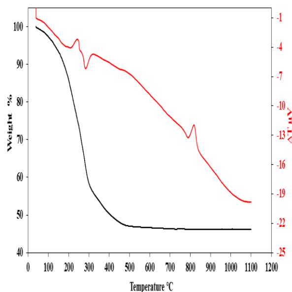
شکل (۱): منحنی آنالیز حرارتی رسوبات خشک شدنی نمونه ZAS_{40}
