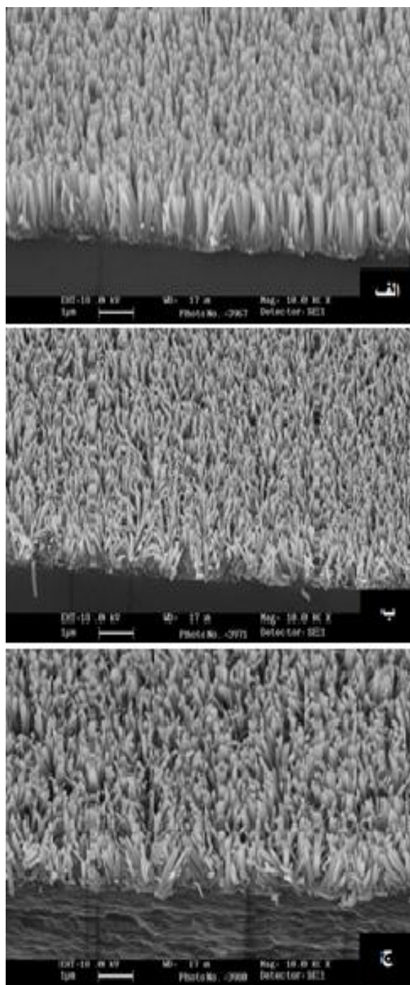
شکل (۶): تصاویر SEM مقطع عرضی نانومیله های ZnO رشد یافته بر روی بذر لایه با ضخامتهای: (الف): ۵۰nm، (ب): ۱۵۰nm و (ج): ۳۰۰nm
