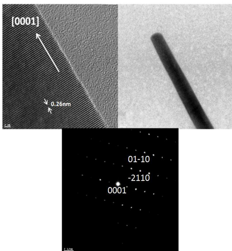
شکل (۸): تصویر HR-TEM نانومیله های ZnO بر روی بذر لایه
