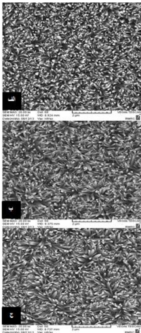
شکل (۷): تصاویر SEM نانومیله سنتز شده بر روی بذرلایه با ضخامت‌های:
