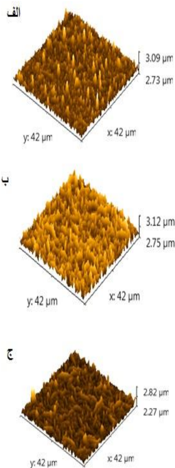
شکل (۳): تصاویر AFM بذرلایه با ضخامت‌های: (الف): ۵۰nm، (ب): ۱۵۰nm و (ج): ۳۰۰nm
