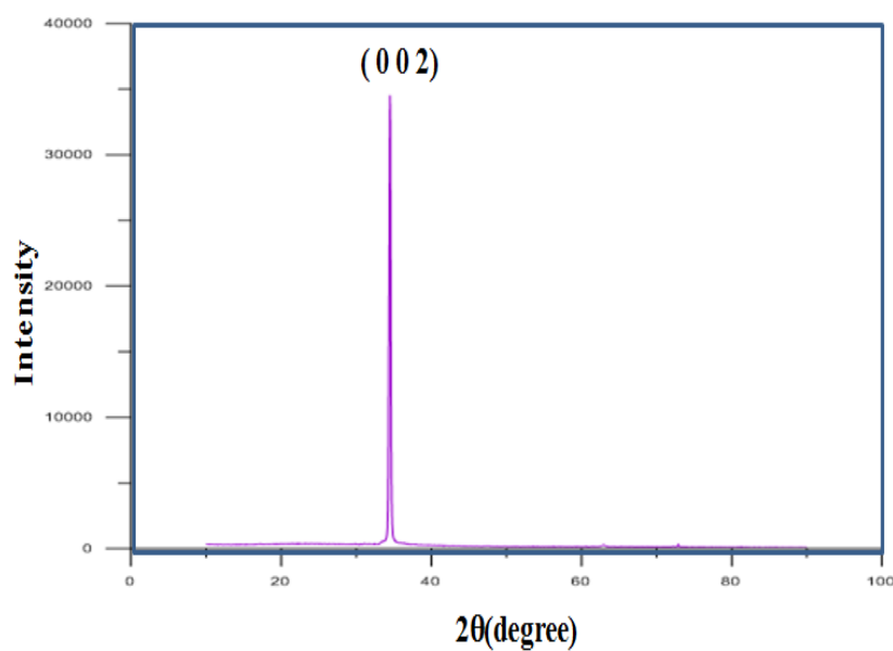
شکل (۹): نتیجه XRD نانومیله های ZnO رشد یافته بر روی بذرایه با ضخامت ۱۵۰nm
