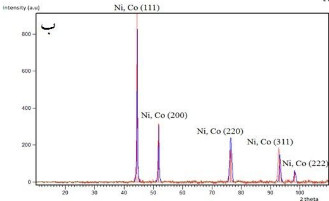
شکل (۱): نتایج پراش اشعه ی ایکس برای: (الف): پوشش نانوکامپوزیتی Ni-Co/SiO 2 و (ب): پوشش آلیاژی Ni-Co
