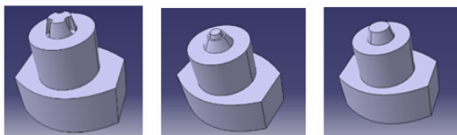
شکل (۱): طرح پین بکار رفته از چپ به راست (مخروطی ناقص - مخروطی ناقص پله دار - تری فلوت)
