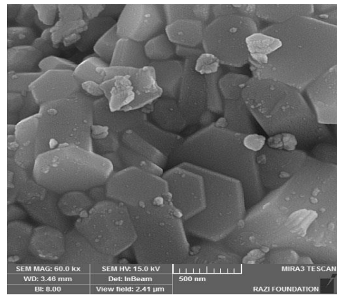
شکل (۵): تصویر SEM نشان دهنده هگزائگونال‌های بزرگتر و ذرات آگلومره کمتر نمونه دوپ شده با کد BZCF
