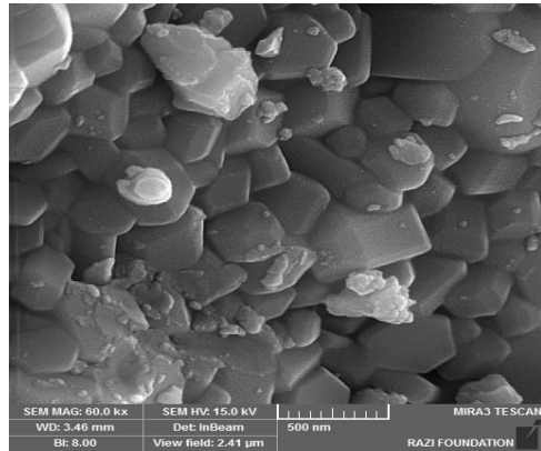
شکل (۴): تصویر SEM نشان دهنده ذرات هگزائگونال برای نمونه دوپ شده با کد BMTF
